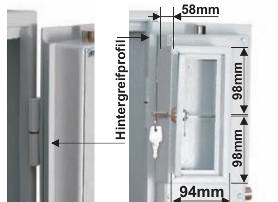
Munitionsfach Innenmasse
