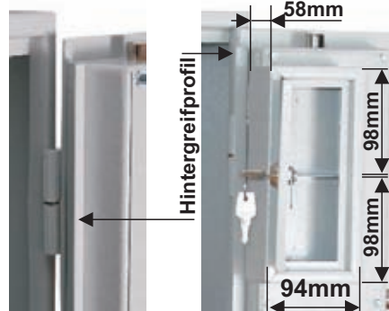
Munitionsfach Innenmasse
