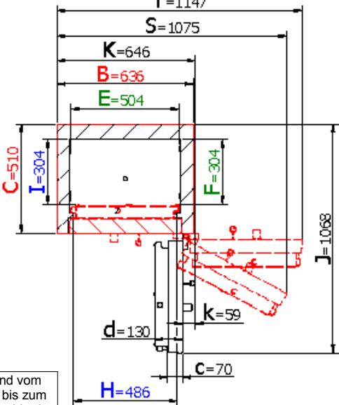
Draufsicht T=1147
