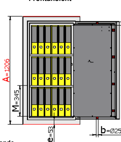
Frontansicht
